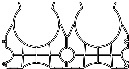
8W34-2 SPACER
