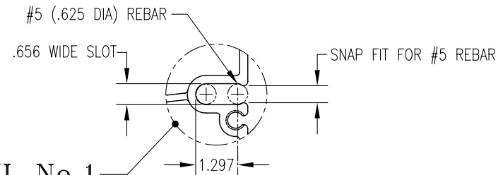
DETAIL No.1 (SCALE: 2.5X)
